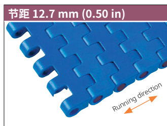
uni M-QNB 强度指数 (聚甲醛)
