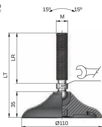
Pie ligero / Light feet Pied léger / Leichtig-Füße
