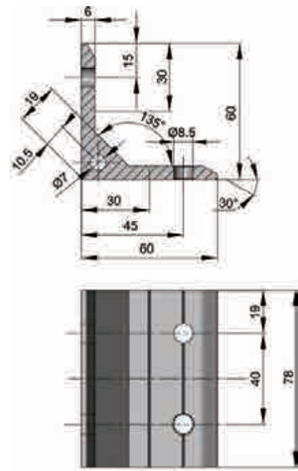
ESCUADRA / BRACKET / ÉQUERRE / WINKEL
