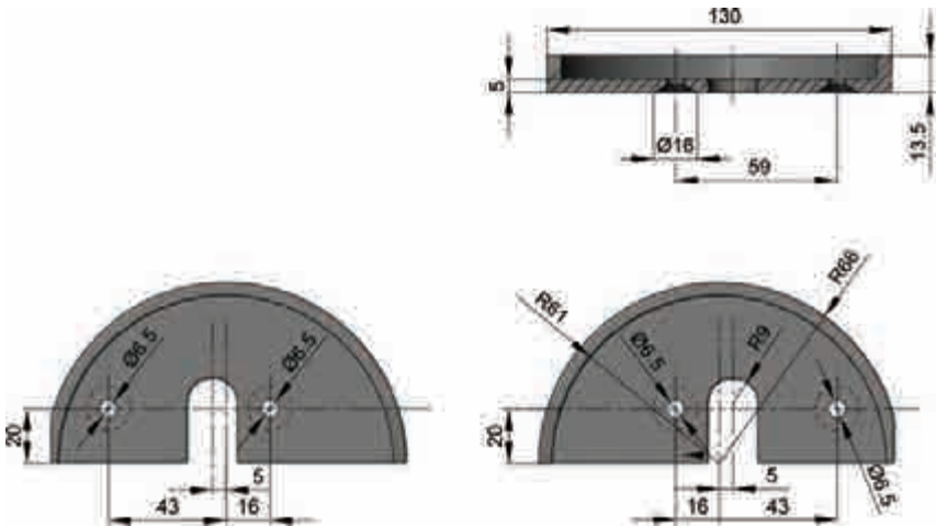
LADO DERECHO TRANSPORTADOR / RIGHT SIDE CONVEYOR / CONVOYEUR CÔTÉ DROIT / FÖRDERER RECHTEHAND
