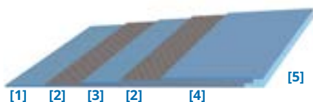
Nastro a due tele con doppia copertura e protezione Amseal ai bordi. [1] copertura inferiore; [2] tessuto; [3] interstrato; [4] copertura superiore; [5] banda Amseal
