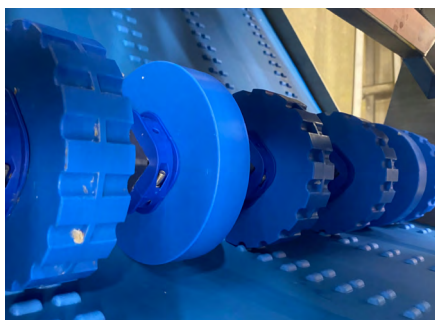
40x40 标准驱动轴
