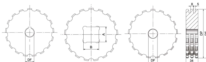
Solid Sprocket
